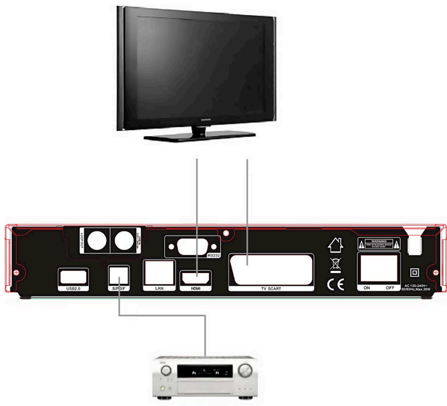
Obrázek 4. Připojení k TV a zesilovači
